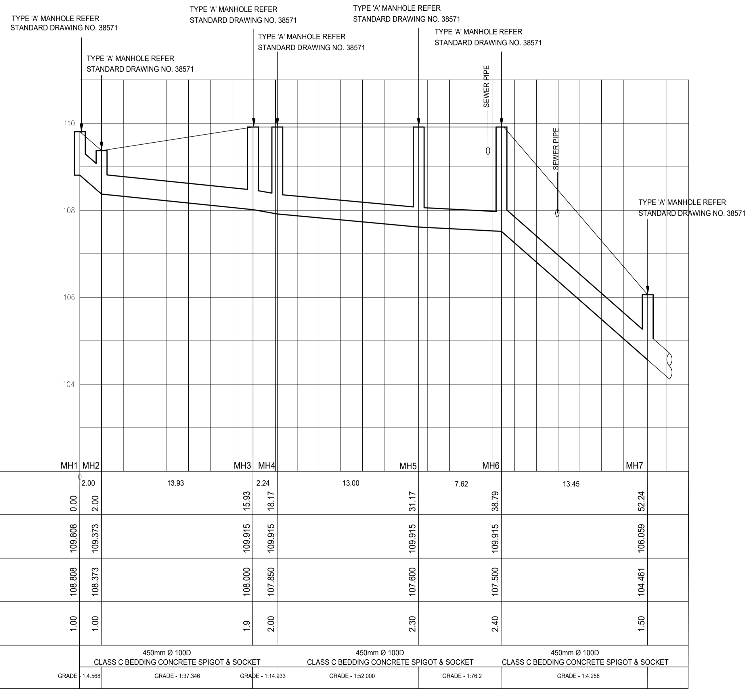
LONGITUDINAL SECTION SCALES - HOR 1:200 VERT 1:50
