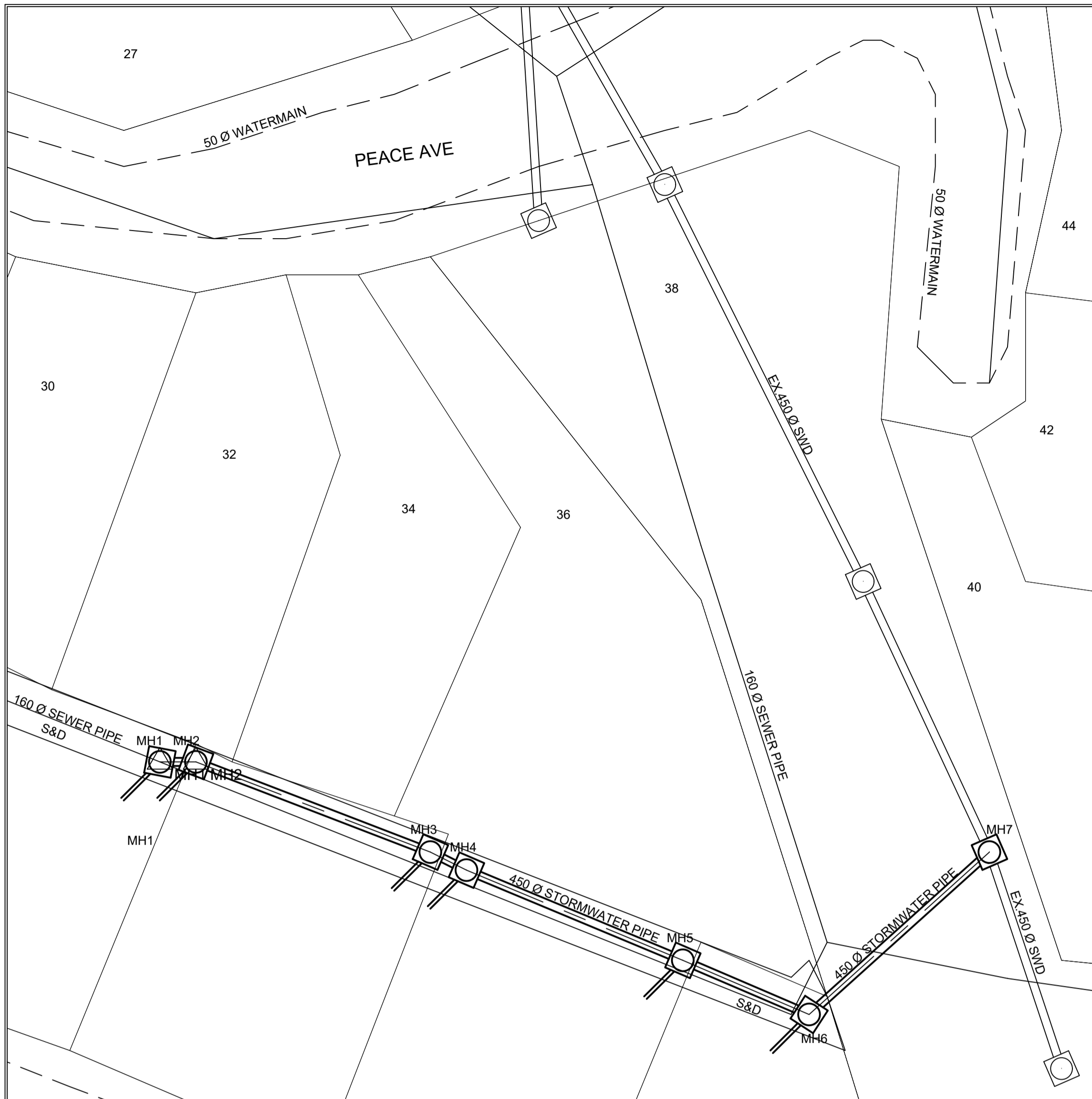
SITE PLAN - PEACE AVE SCALE 1:200
